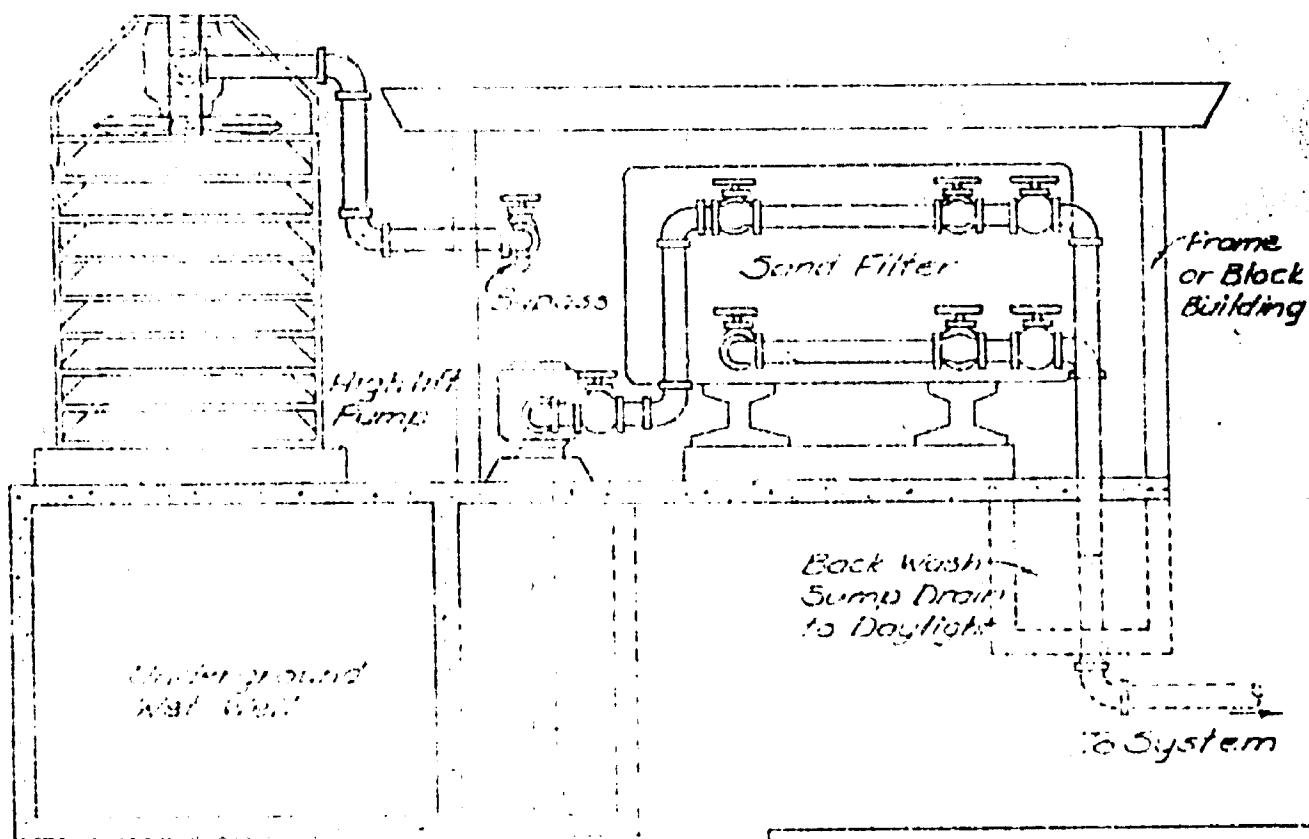
ELEVATION
